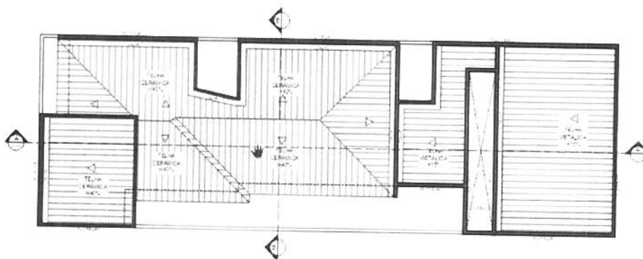
Fig 1 – Planta da cobertura.
