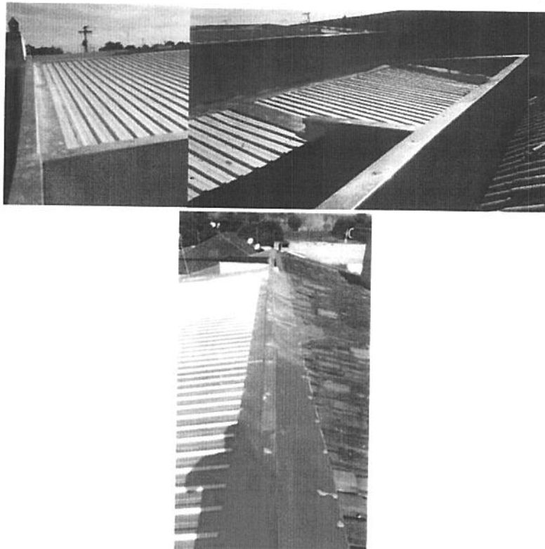
Fig.3 – Instalação de calhas e rufos.
